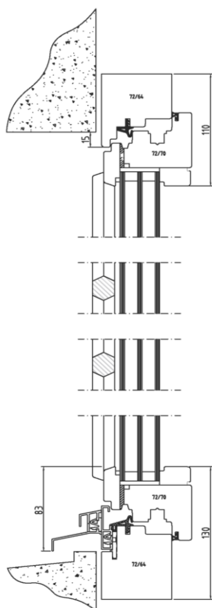
Coupe A-A
