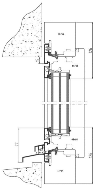
Coupe A-A
